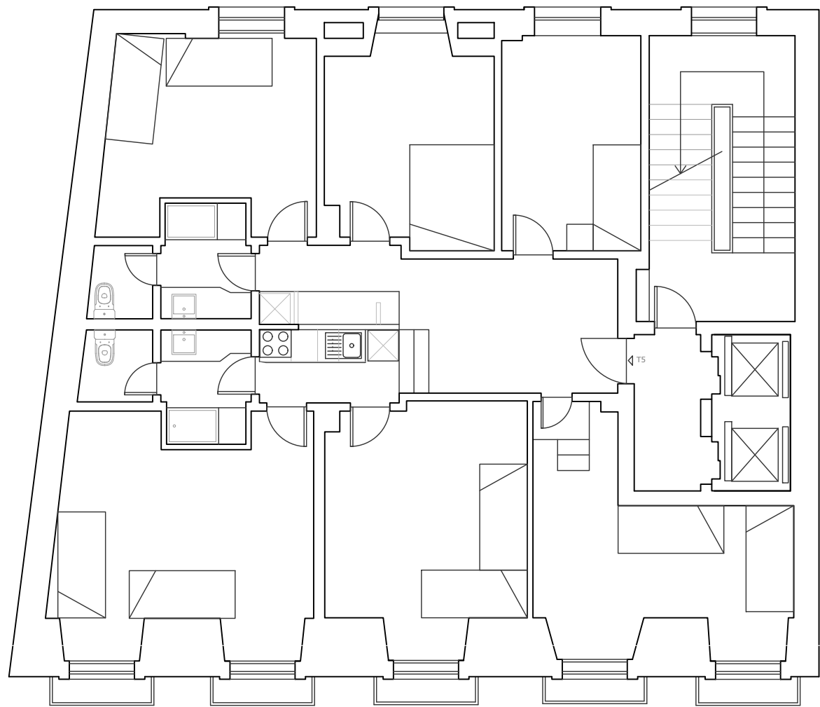
Piso 2
