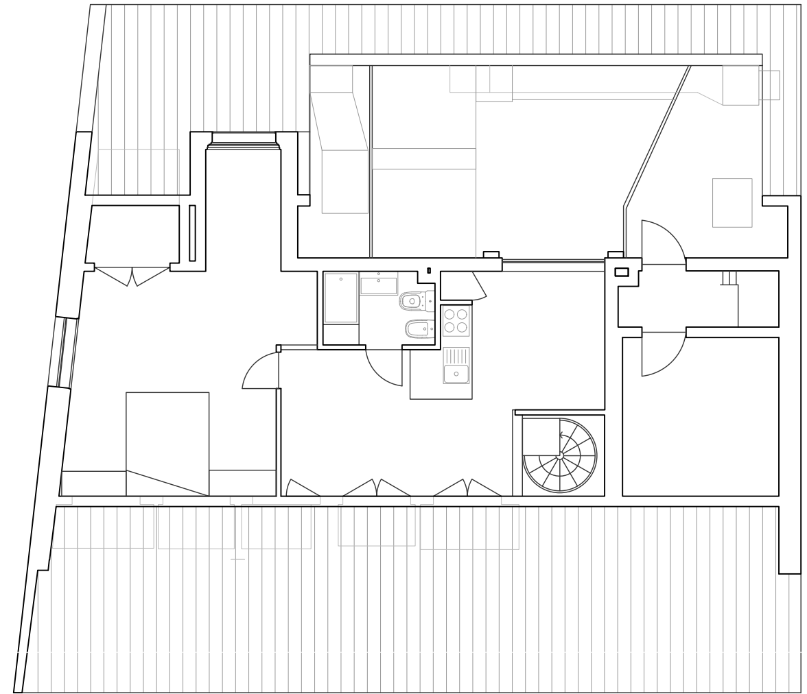
Piso 5 - Mezzanine
